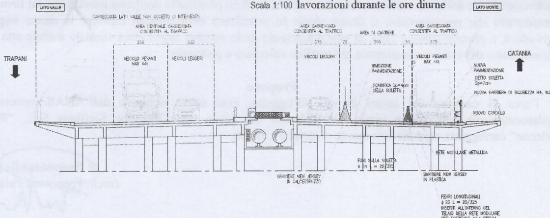
FASE 4: rinforzo estradosso mediano Scala 1:100 lavorazioni durante le ore diurne
