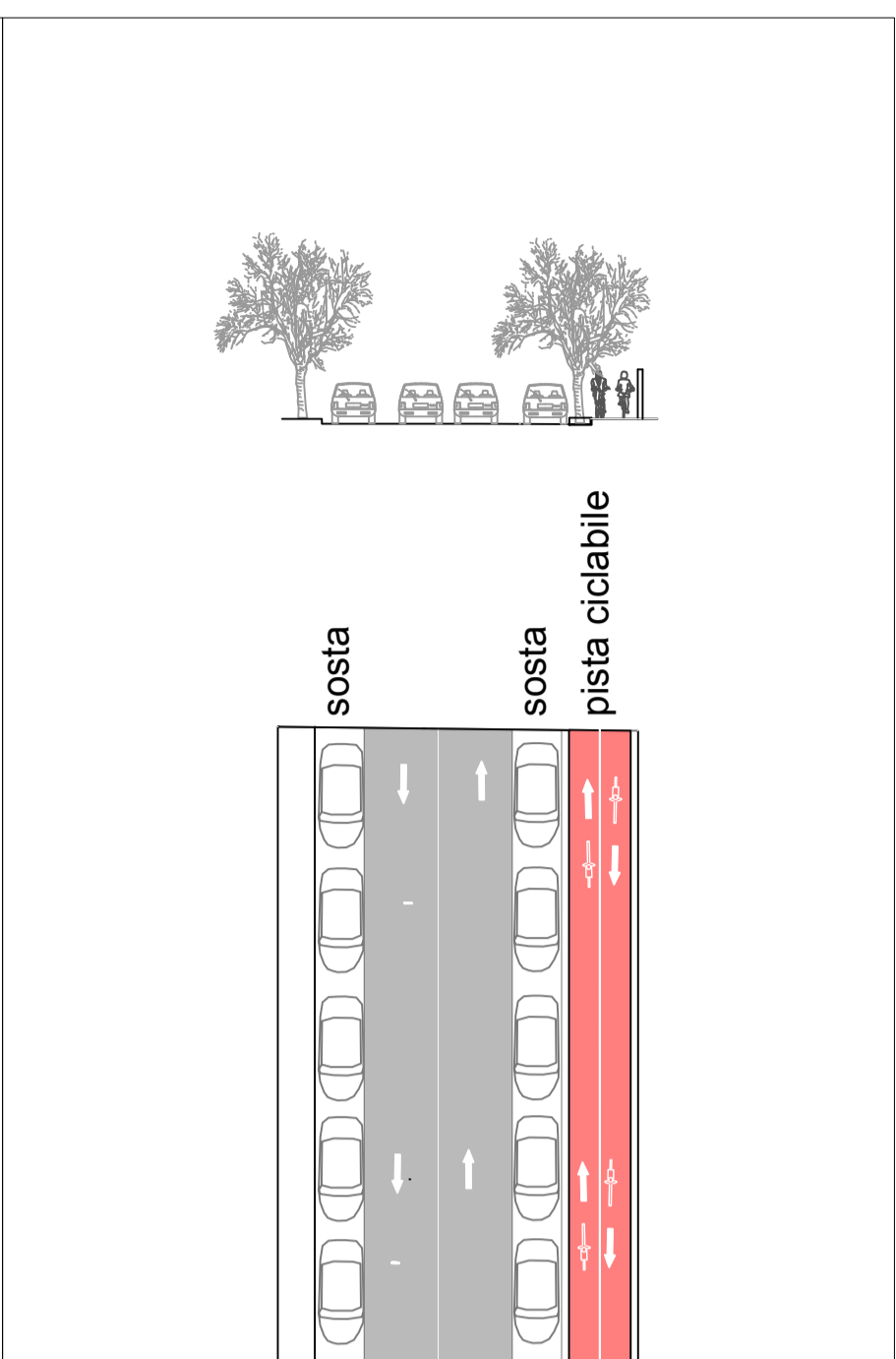
SEZIONE TIPO
